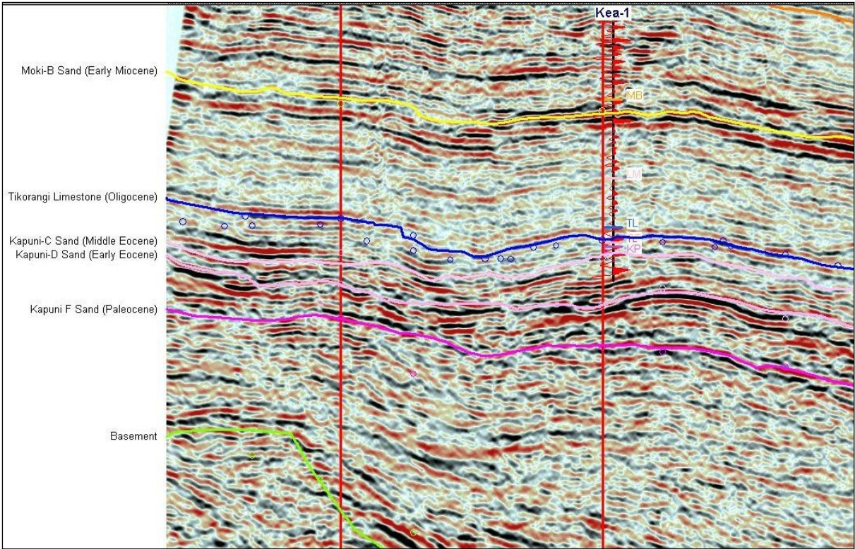
Seismic Section – Kea-1
